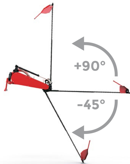
Maximum inclination during working from +90° to -45°. Inclinaison maximale pendant le travail de +90° à -45°.
