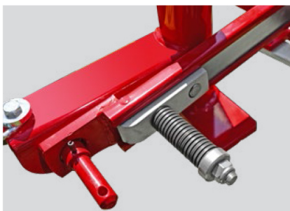
Safety release in case of collision with obstacles. Déclenchement de sécurité en cas de collision avec des obstacles.
